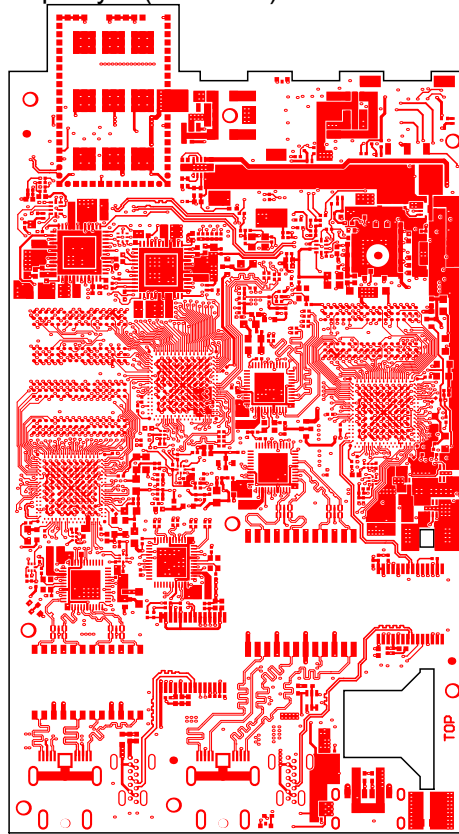
Top Layer (Scale 1:1)
