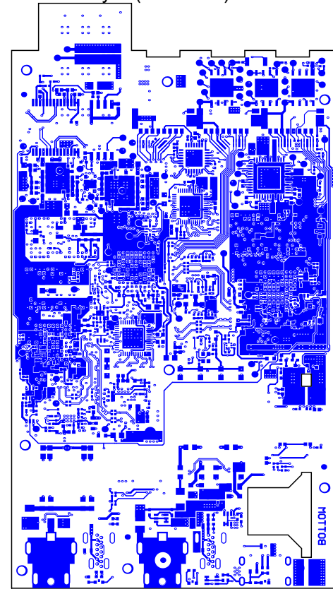
Bottom Layer (Scale 1:1)
