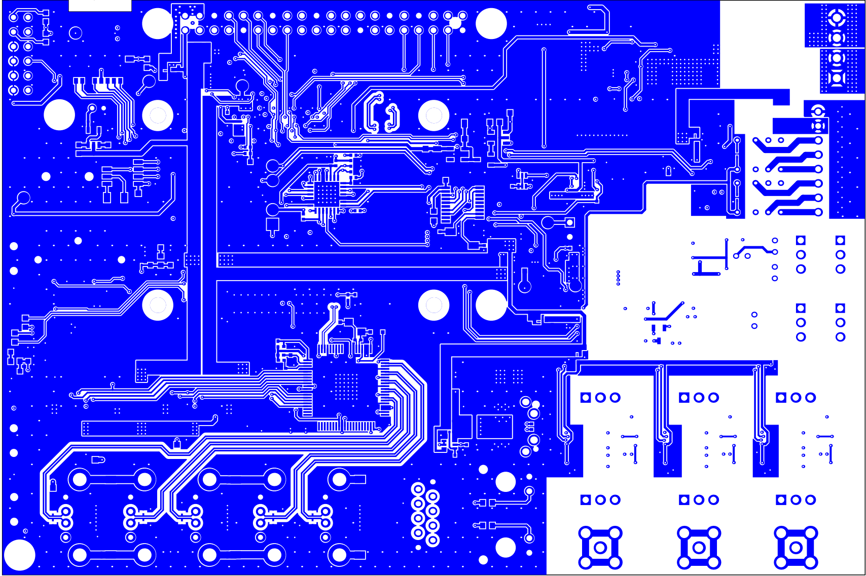
Bottom Layer (Scale 3:2)
